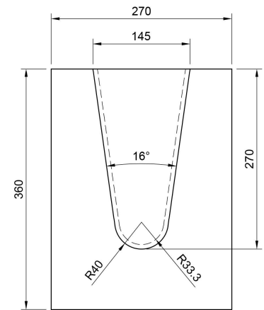
LT180 Dimensions
