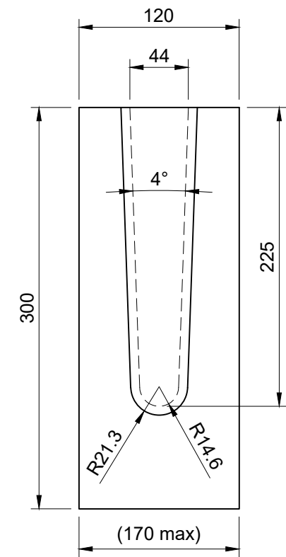
LT060 Dimensions
