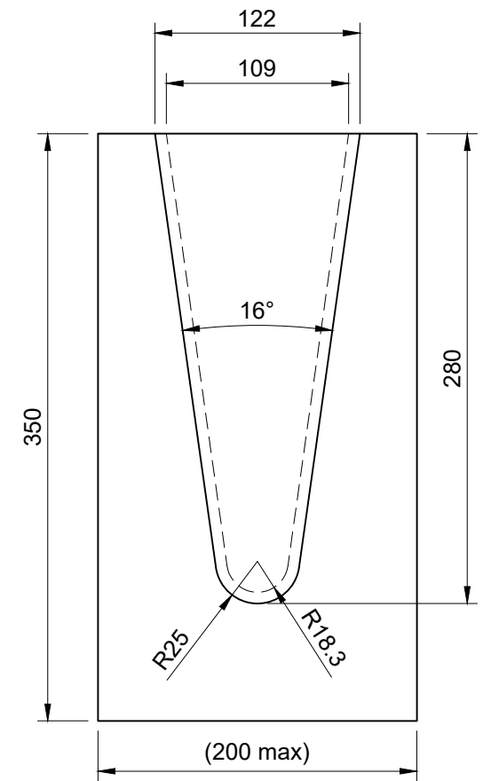
LT120 Dimensions
